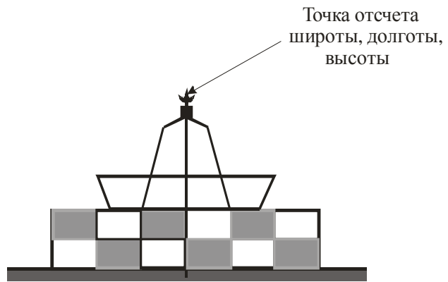
Рис. 8. Точки геодезической привязки DVOR.
